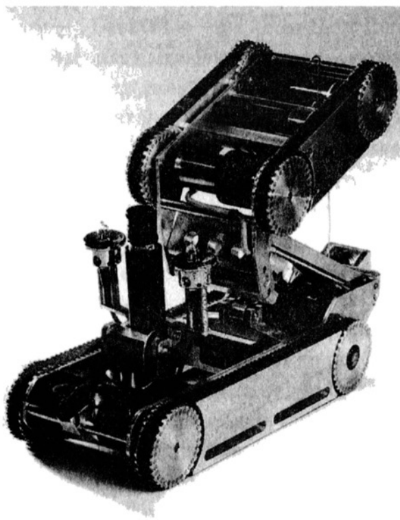
Робот URPAUT, сконструиро- ванный Рудольфом Гантенбрин- ком
